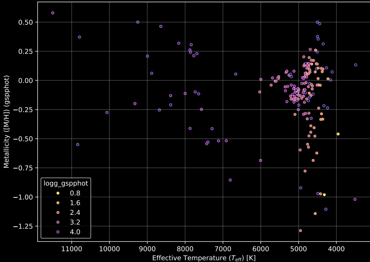
APOGEE DR17 Field: [150-16] Stellar Population Parameters (n= 185)
